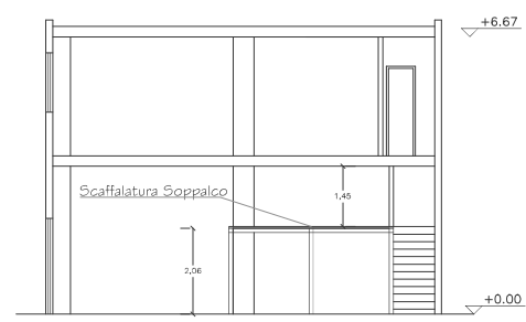
SEZIONE A - A'
